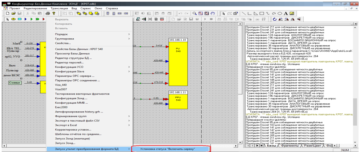
Рис. 3. Автоматическая установка статуса «Включить сирену»
